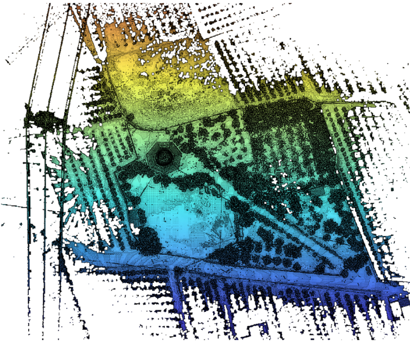
Imagen 1. Vista area de la nube de puntos Image 1. Point cloud area view
