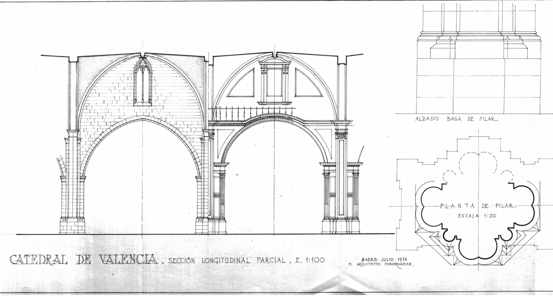
Imagen 5. Levantamientos de Alejandro Ferrant para el descubrimiento del gótico en la segunda mitad del s. XX.
