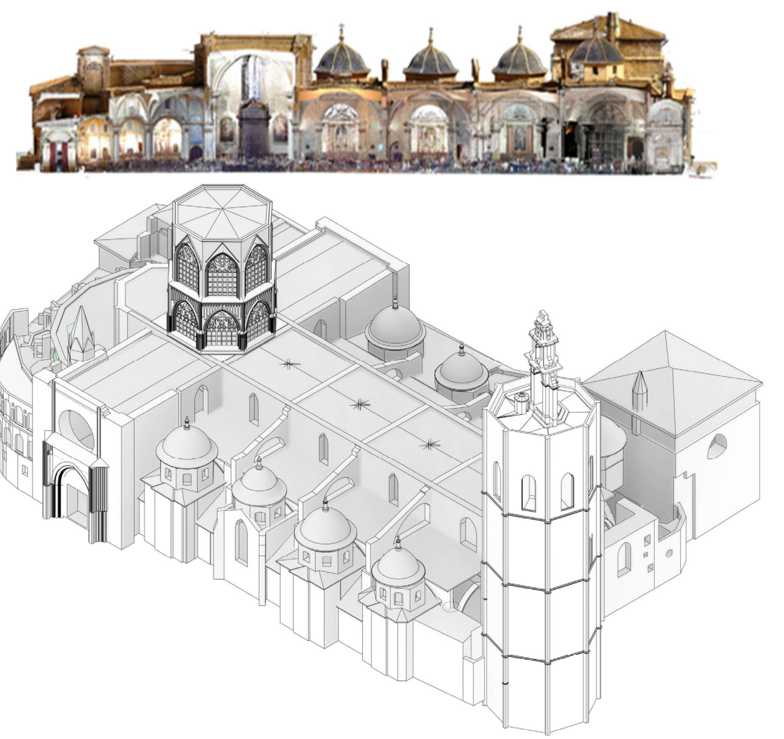
Imagen 6. Levantamiento actual de la Catedral con tecnología escaner 3D (TLS).
