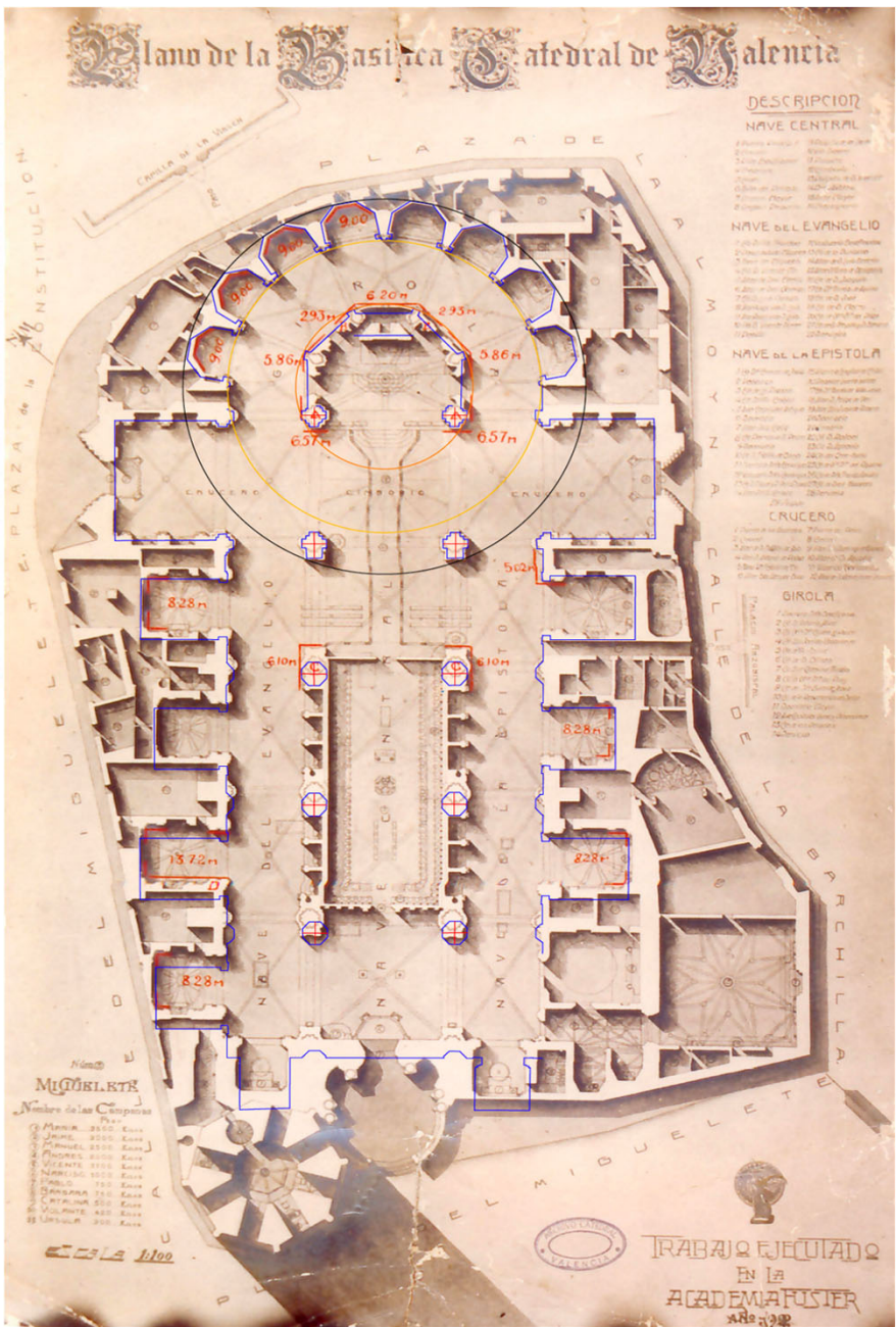
Imagen 4. Levantamiento de la planta por la Academia Fuster, 1922. En azul, el levantamiento actual. Se aprecia el error del levantamiento.
