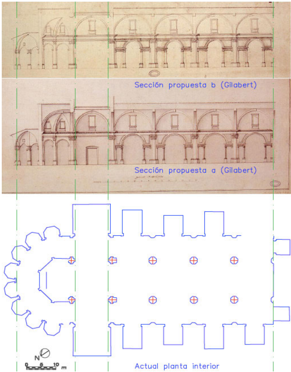
Imagen 3. Propuesta de Gilbert para la renovación de la Catedral (s. XVIII) sobre el levantamiento actual
